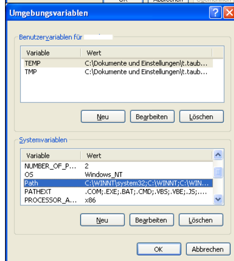
Abbildung: Umgebungsvariablen
